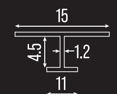
Verbinder 4 mm
