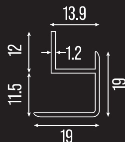
Buitenhoek 11mm
